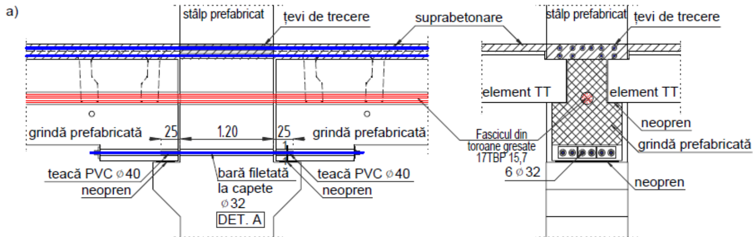
SECȚIUNE 1-1
