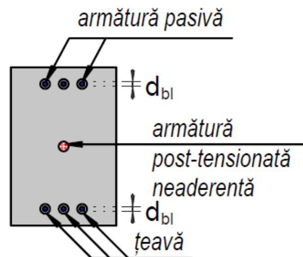
SECȚIUNE 1-1
