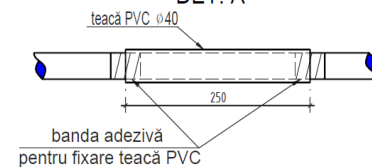
DET. A
