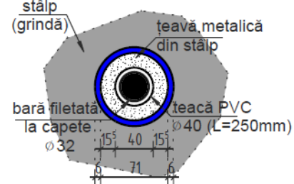
SECȚIUNE 1-1
